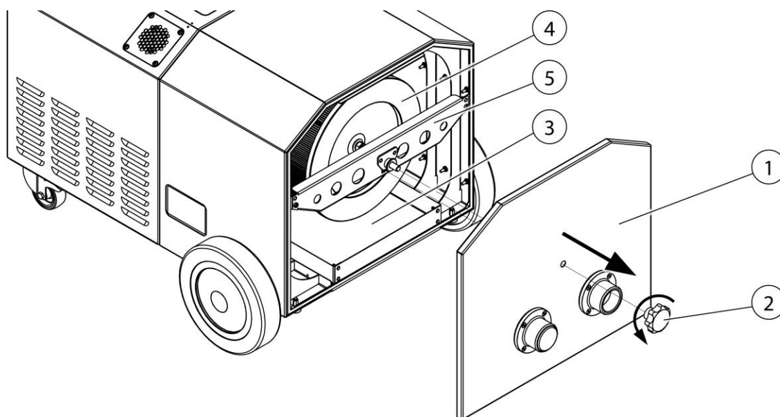
Fig. 6: Acesso ao recipiente coletor de pó
